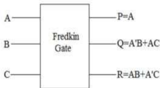
Fig. 3: FREDKIN GATE
