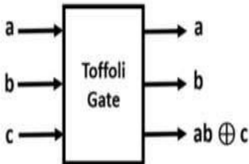
TOFFOLI GATE
